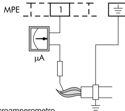
Collegamento microamperometro
