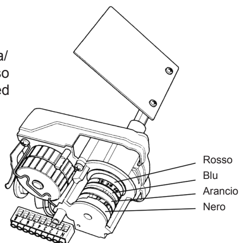
Servocomando
