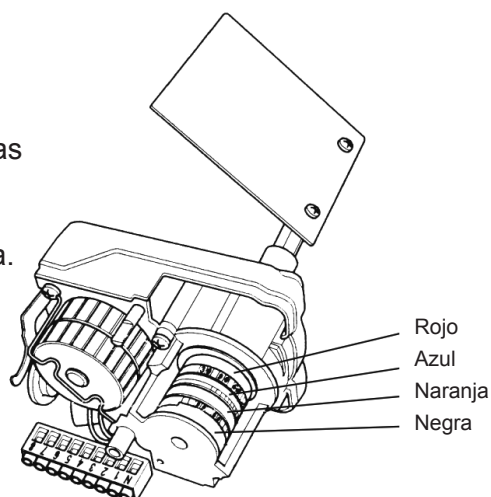
Servomando
